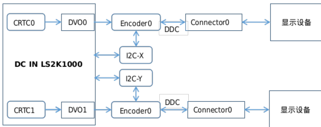
图 2-2: 非透明输出类型的显示编码器的显示连接方案
